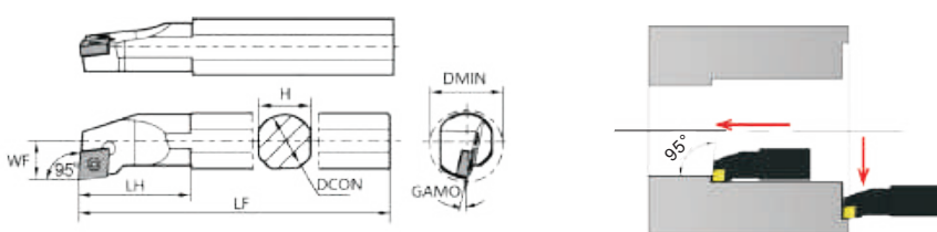
S□□-SCLCR/L KAPR:95°
