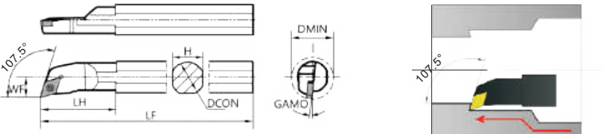
S□□-SDQCR/L KAPR:107.5°
